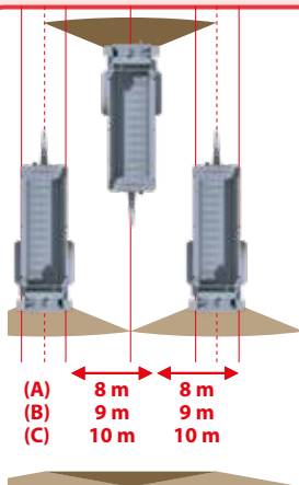
Szeroka naprzemienna praca wałków (szerokość zależna od materiału): (A) 8 m (standard) (B) 9 m zębami łopatkowymi (C) 10 m z tarczami rozrzucającymi
